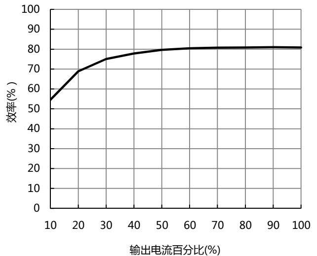
图 6. B0505S-1W 效率 vs 输出负载 (标称输入)
