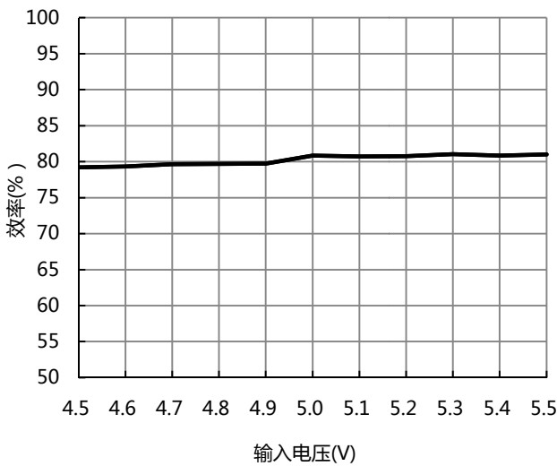
图 5. B0505S-1W 效率 vs 输入电压 (满载)
